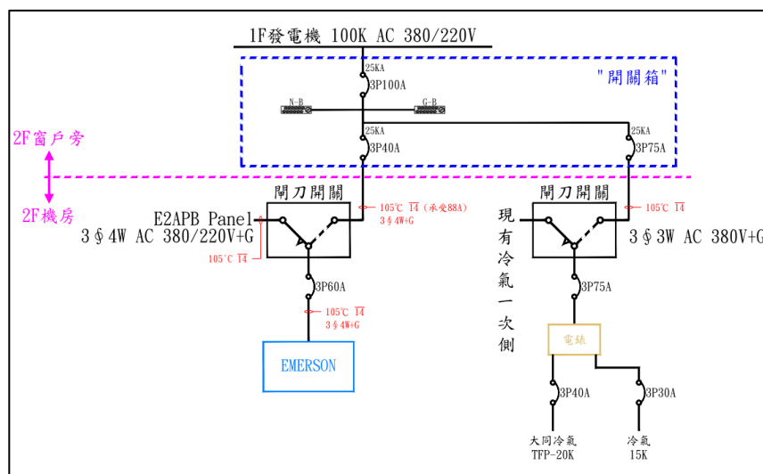
(圖十五)、 第二迴路發電機-配電圖
