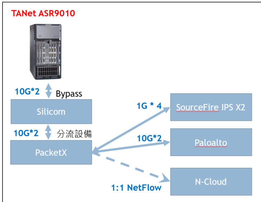
(圖十)、資安架構圖
